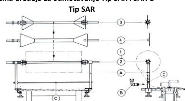
Šema uređaja za odmotavanje Tip SAR i SAR-D
